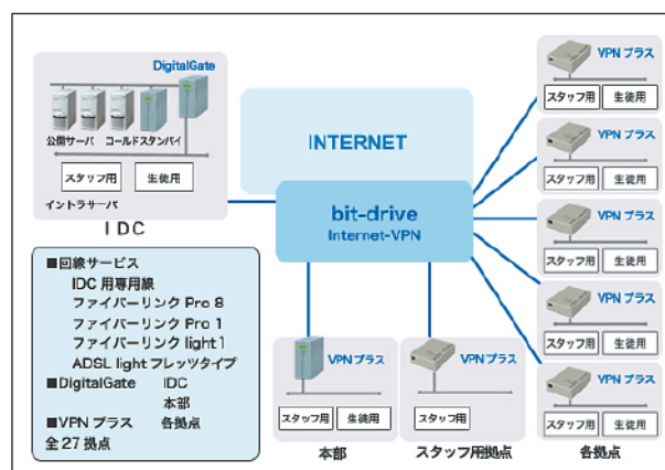
<株式会社バンタンさま ネットワークイメージ図>
